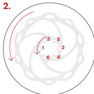
Hamulce tarczowe – Trexx Disc
