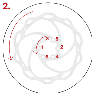
Disk kočnice – Trexx Disc
